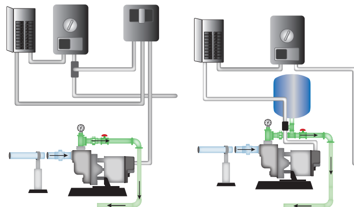
Conmutador de arranque de la bomba
