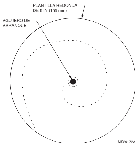
Fig. 6. Corte para la abertura del desviador.
