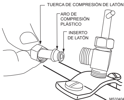
Fig. 9. Instalación de la tubería de alimentación.
