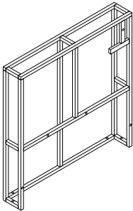
Right frame (1 pc)
