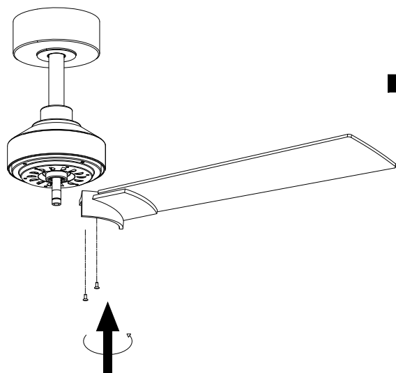
Installation fan blade diagram
