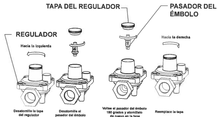
Fig. 7 - Conversión del regulador
