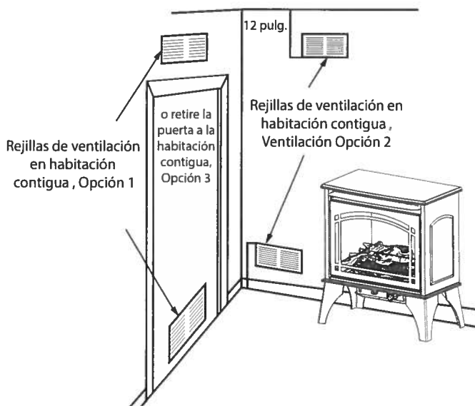
Fig. 4 - Aire de ventilación desde el interior del edificio
