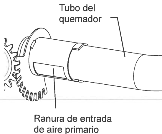
Fig. 24 - Ranura de entrada de aire primario en el tubo del quemador
