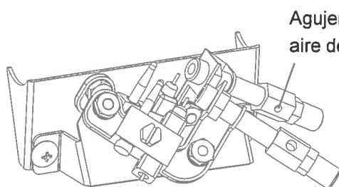
Fig. 24 - Ranura de entrada de aire primario en el tubo del quemador
