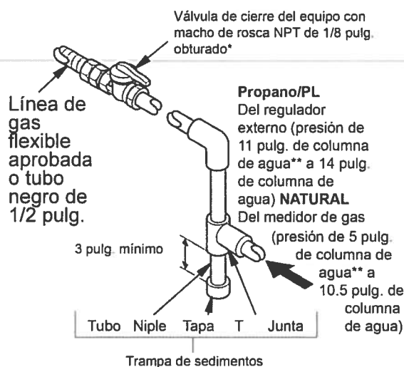
Fig. 10 - Conexión del gas
