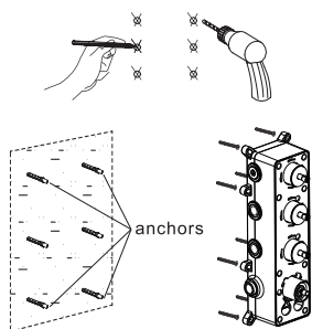
(Pared de concreto)
