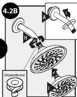
4.2B Regadera con junta de bola de metal
