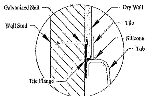
Non Integral Flange
