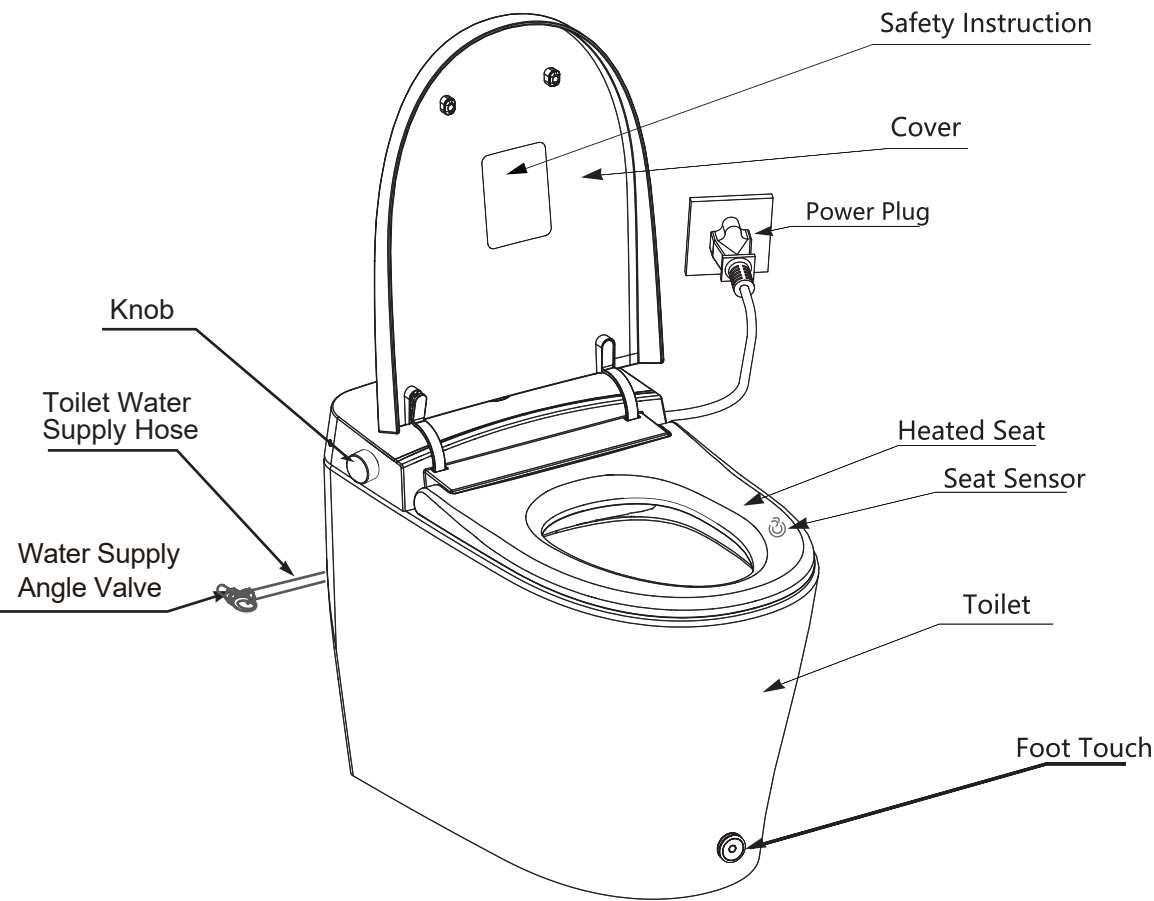
Knob
