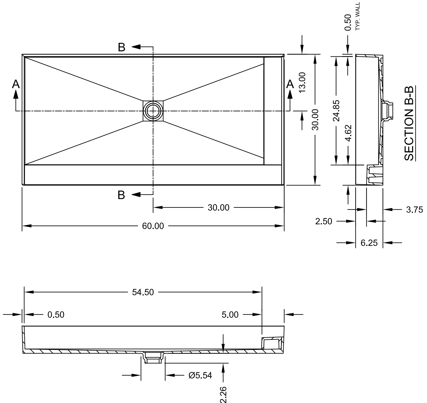
SECTION A-A
