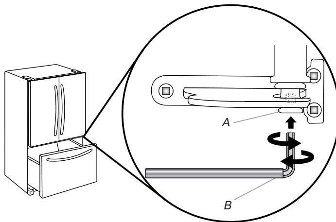
A. Pasador de la bisagra inferior B. Llave hexagonal en L de \frac{1}{8} "
