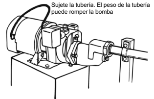
Figura 4B: sostenga de forma independiente toda la tubería fijada a la bomba
