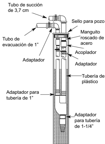
Figura 3: eyector para pozo profundo
