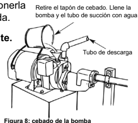
Figura 8: cebado de la bomba
