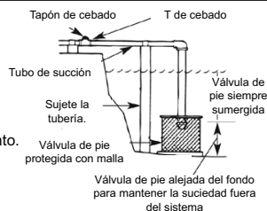
Figura 5C: Instalación en el lago
