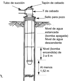
Figura 5A - Instalación para el pozo excavado/entubado
