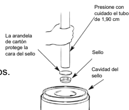
Figura 12: si es necesario, presione con un cartón y un tubo
