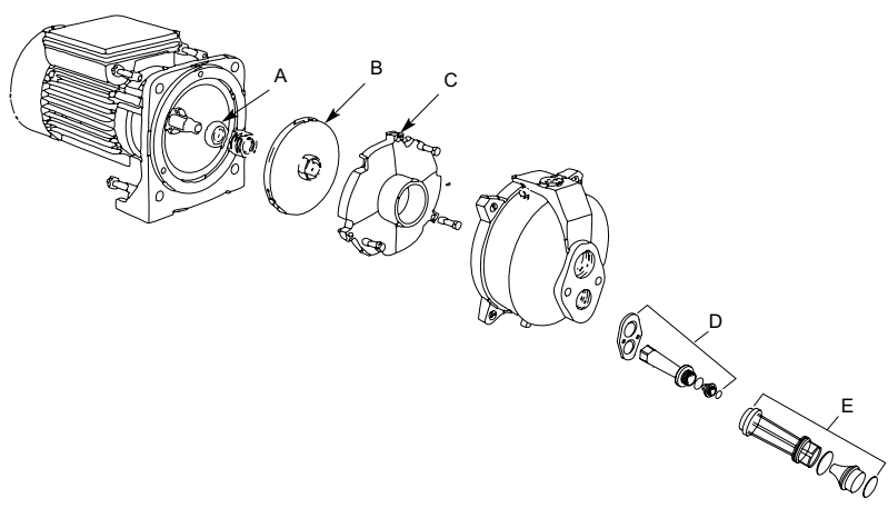
Figura 13: ilustración de las piezas de reparación para las bombas de chorro convertibles
