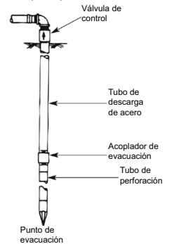
Figura 5B - Instalación del punto de descarga
