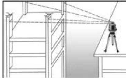
Instalación de piso de cemento
