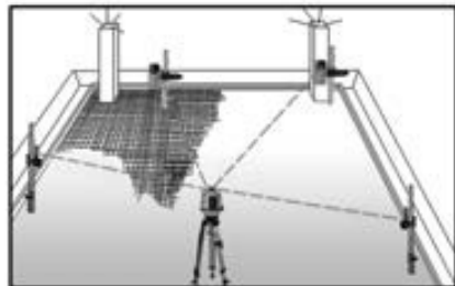
Escuadrado y nivelación
