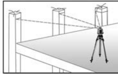
Construcción de muros o cimentación
