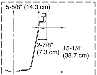
Drain Detail Détails du drain Detalle del desagüe
