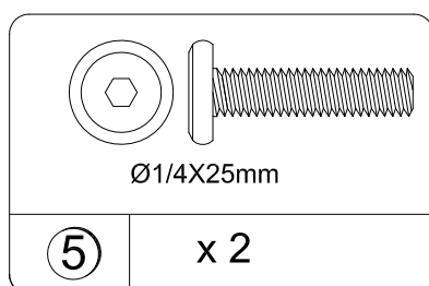
Bolt TSF1416
