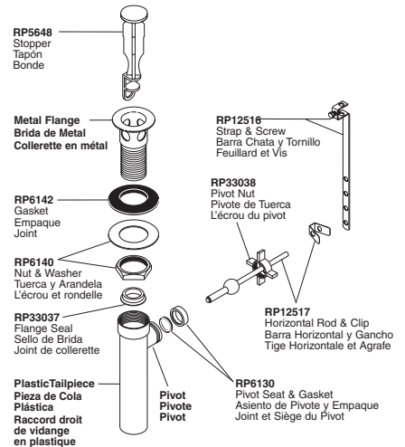
RP38958 Pop-Up Assembly Less Lift Rod Ensamble del Desague Automático sin la barra para alzarlo Renvoi mécanique sans la tirette
