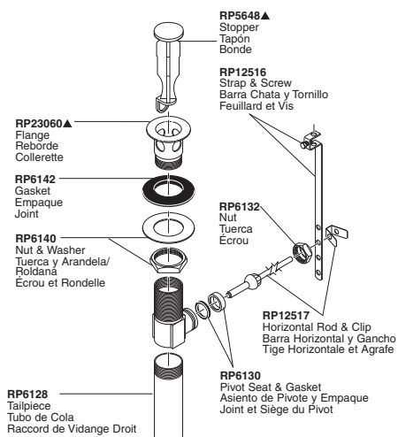
RP26533▲ Metal Pop-Up Assembly Less Lift Rod Ensamble de Metal del Desague Automático Menos la Barra de Alzar Renvoi Mécanique en Métal Sans la Tige de Manoeuvre
