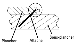
ATTACHE CORRECTEMENT ENFONCÉE
