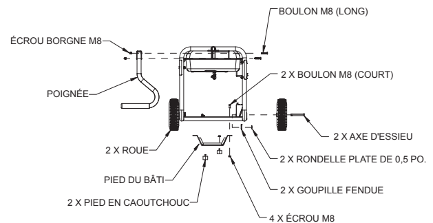
Schéma 1 – Roue et poignée
