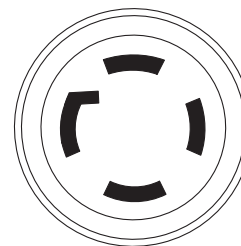
Figura 6 - Receptáculo de 120/240 VAC, 30 Amp
